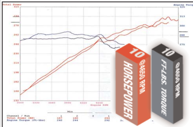
Dyno Chart: 2001 BMW M5 (E39)
